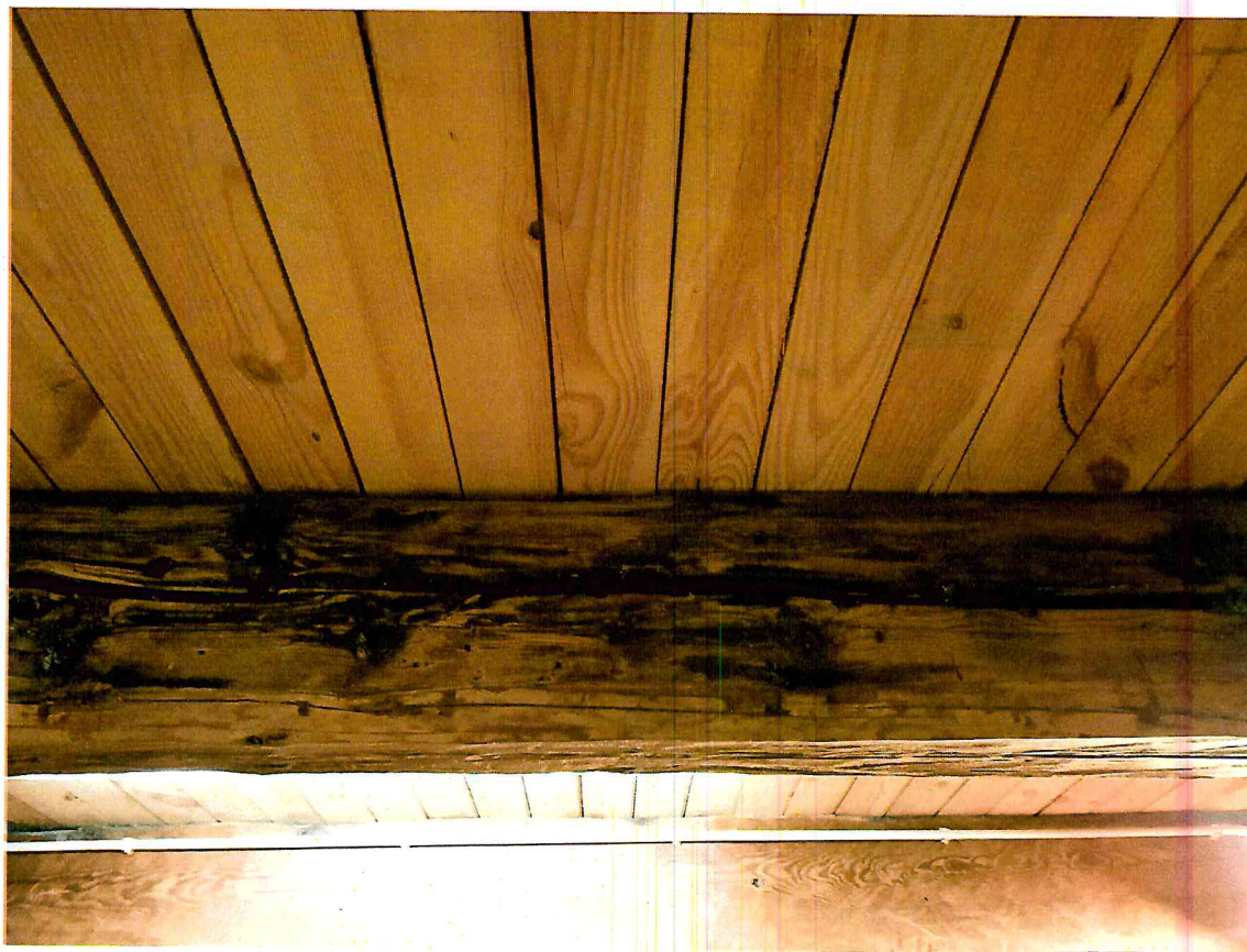
FF-17. Medienos įtrūkimas.
