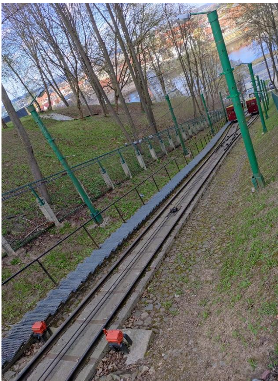
Nr. 3 Pavadinimas Aleksoto funikulieriaus statinių komplekso kelias su įranga Fotografavo Skaistė Dikaite ir Kamilė Muravjovaitė Data 2021-04-28
