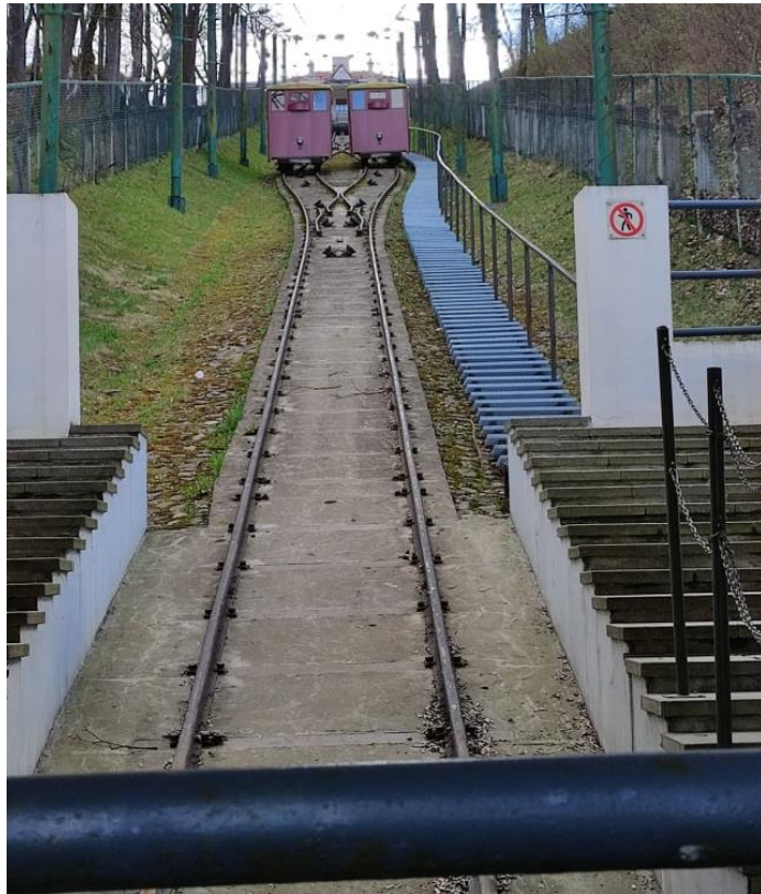
Nr. 1 Pavadinimas Aleksoto funikulieriaus statinių komplekso kelias su įranga Fotografavo Skaistė Dikaite ir Kamilė Muravjovaitė Data 2021-04-28
