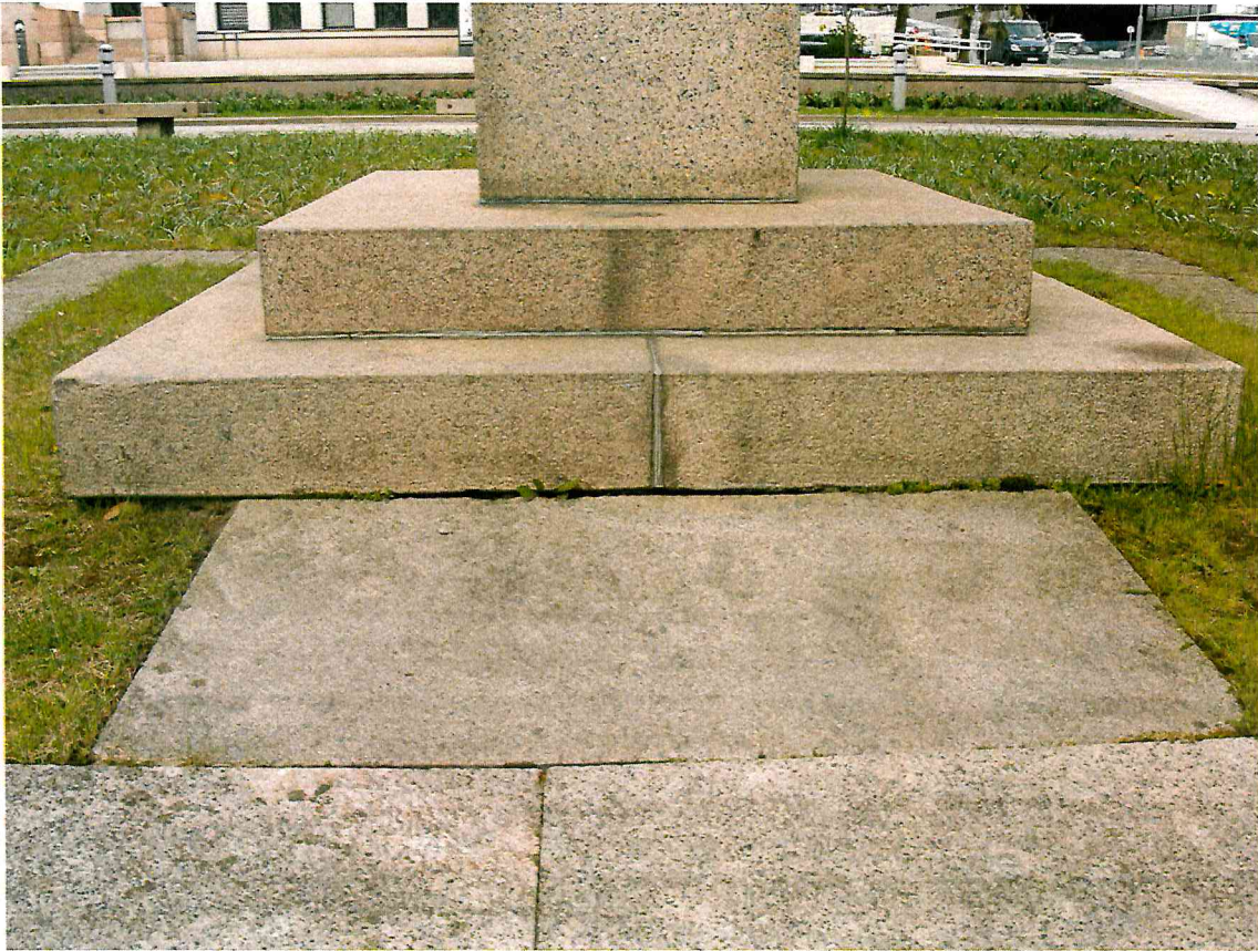
7 pav. Tarp cokolio apatinio laipto ir žemės paviršiaus yra susiformavęs tarpas. Pasmukusi priekinė granito plokštė
