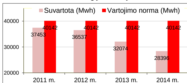
107 pav. Šilumos energijos naudojimo tendencijos bendrojo ugdymo mokyklose
