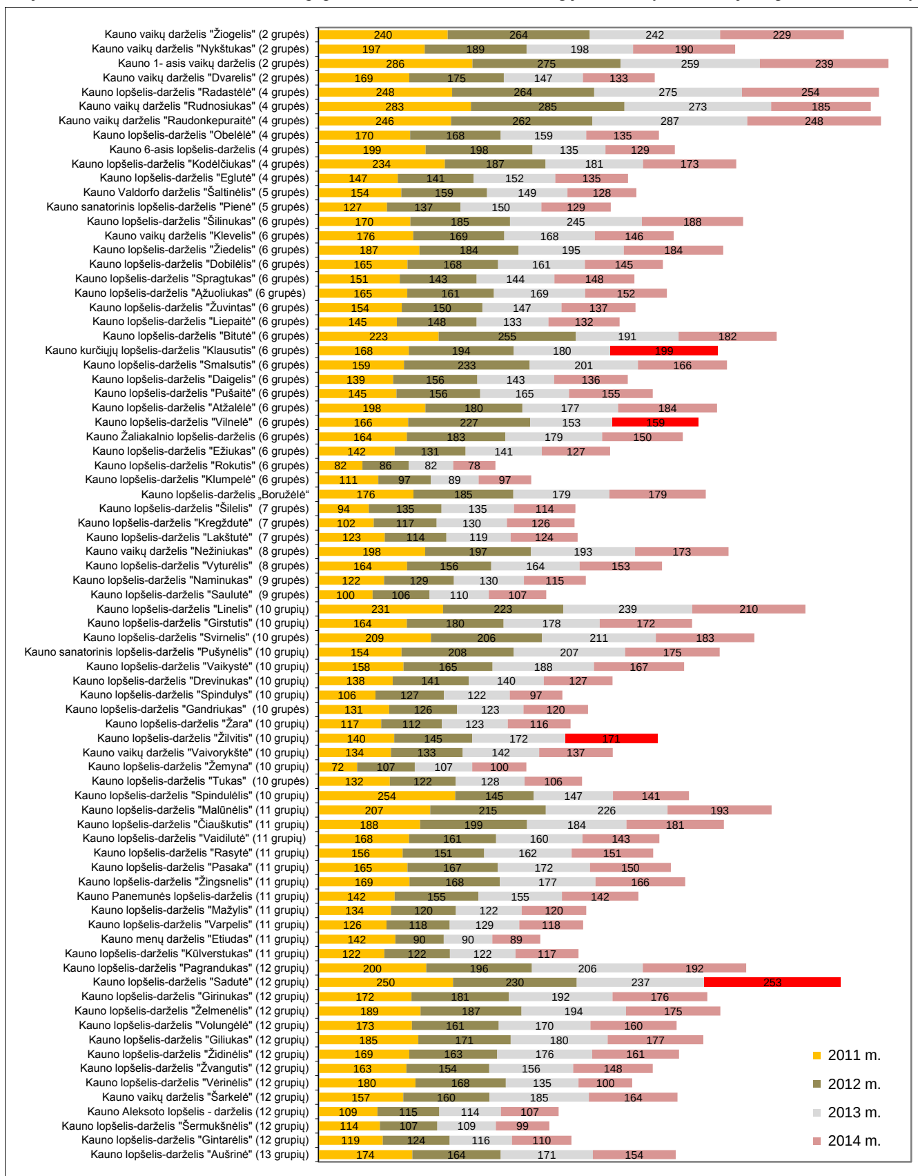
114 pav. Šilumos energijos vartojimo kiekis ikimokyklinio ugdymo įstaigose (Kwh/m 2 ).
