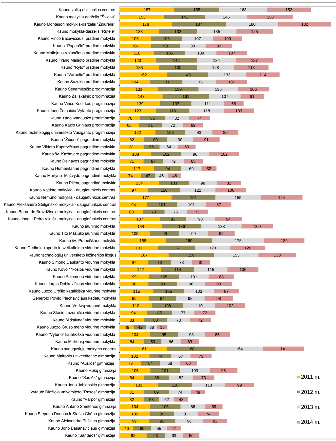
115 pav. Šilumos energijos vartojimo kiekis bendrojo ugdymo mokyklose (Kwh/m 2 )
