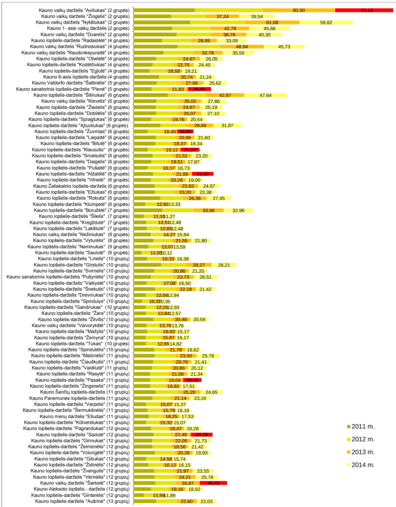
113 pav. Elektros energijos vartojimo kiekis ikimokyklinio ugdymo įstaigose (Kwh/m 2 )
