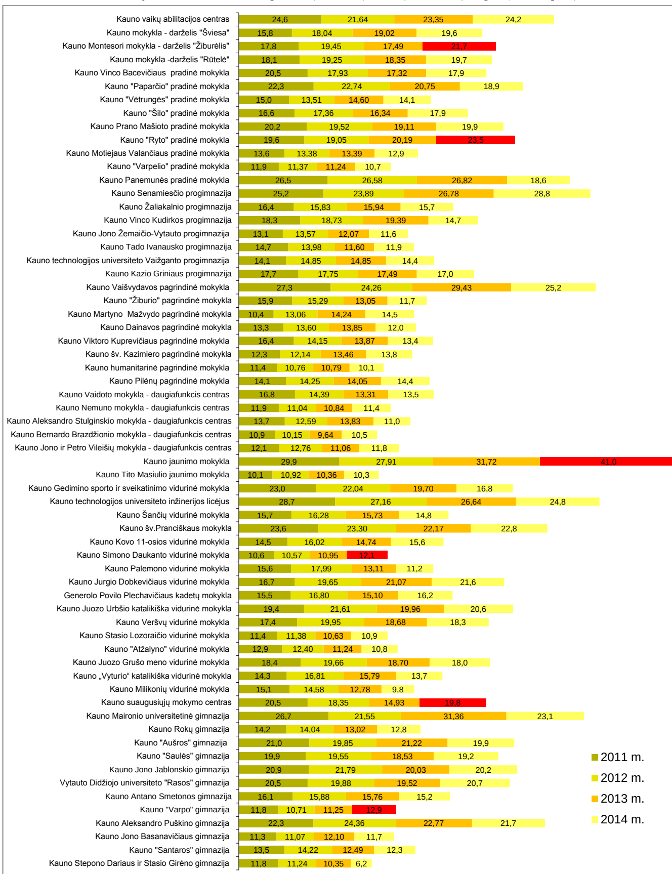
112 pav. Bendrojo ugdymo mokyklose elektros energijos kiekis, tenkantis bendrojo ploto vienetui (Kwh/m 2 )
