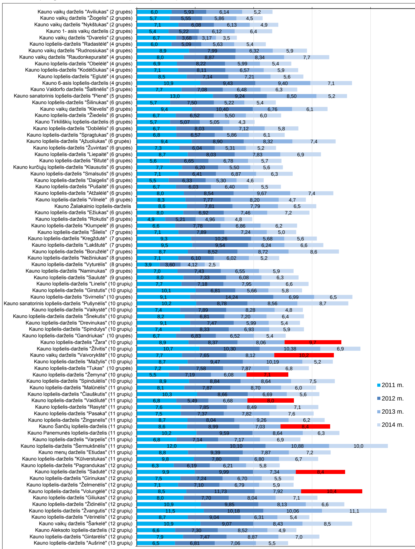
111 pav. Vandens vartojimo kiekis ikimokyklinio ugdymo įstaigose ( m^3/\text{žmogui} ).
