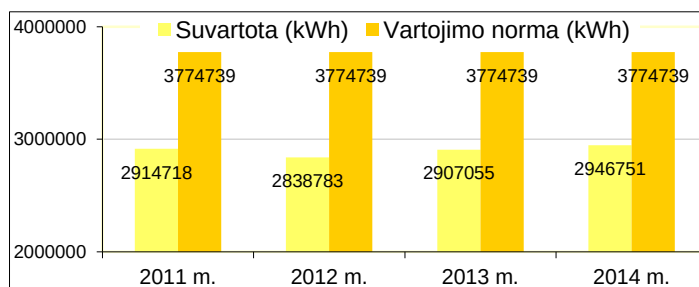
105 pav. Elektros energijos naudojimo tendencijos ikimokyklinio ugdymo įstaigose
