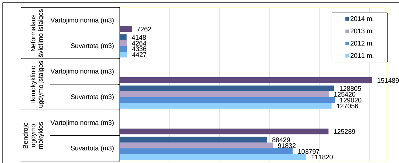
103 pav. Vandens vartojimo tendencijos švietimo įstaigose pagal tipus
