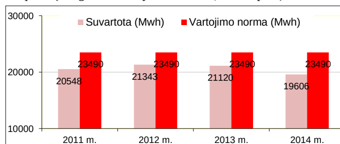
108 pav. Šilumos energijos naudojimo tendencijos ikimokyklinio ugdymo įstaigose
