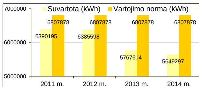
104 pav. Elektros energijos naudojimo tendencijos bendrojo ugdymo mokyklose
