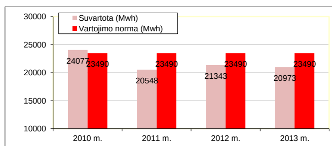
109 pav. Šilumos energijos naudojimo tendencijos ikimokyklinio ugdymo įstaigose
