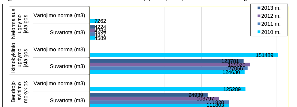
104 pav. Vandens vartojimo tendencijos švietimo įstaigose pagal tipus
