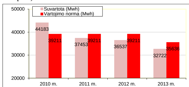
108 pav. Šilumos energijos naudojimo tendencijos bendrojo ugdymo mokyklose
