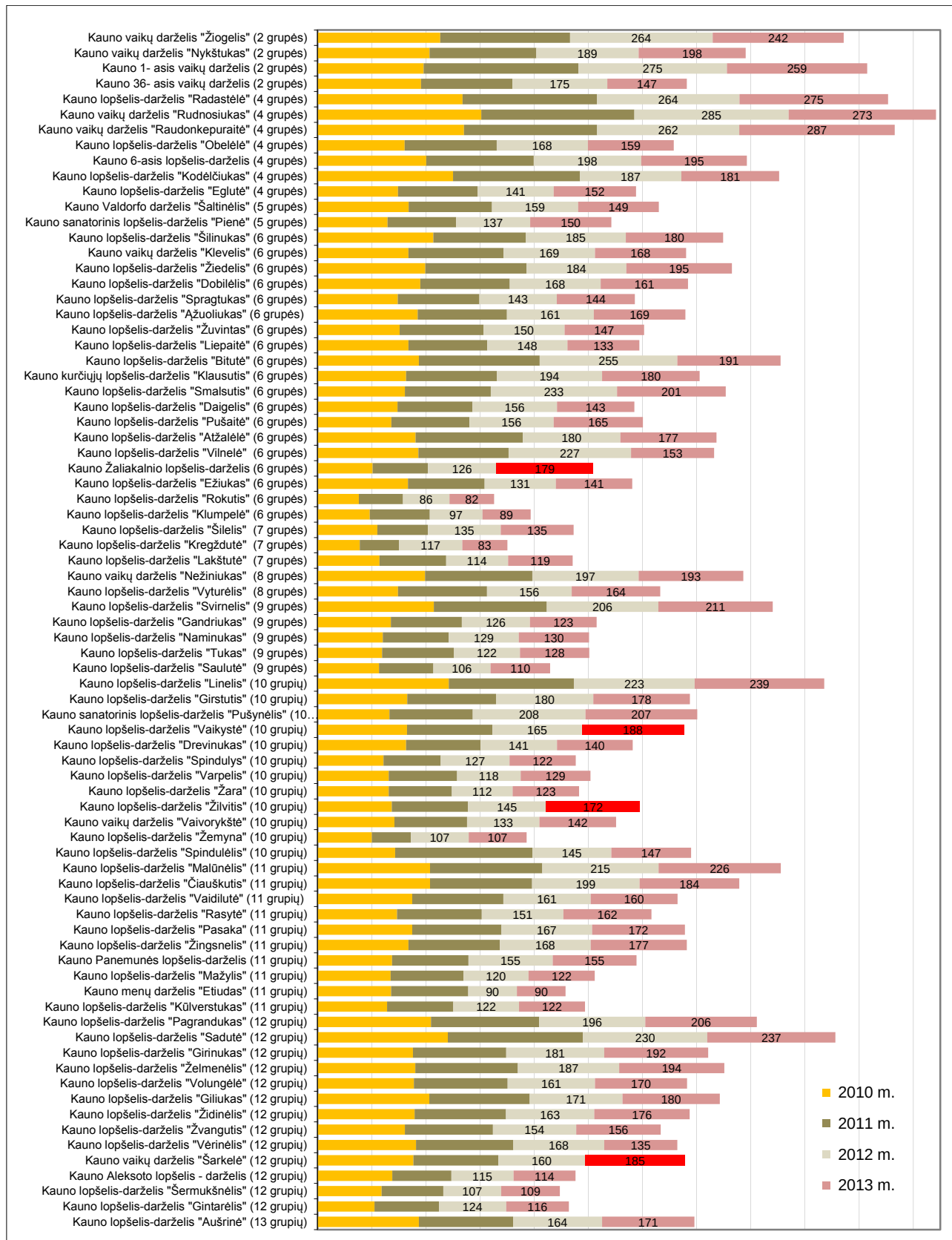
115 pav. Šilumos energijos vartojimo kiekis ikimokyklinio ugdymo įstaigose (Kwh/m²).
