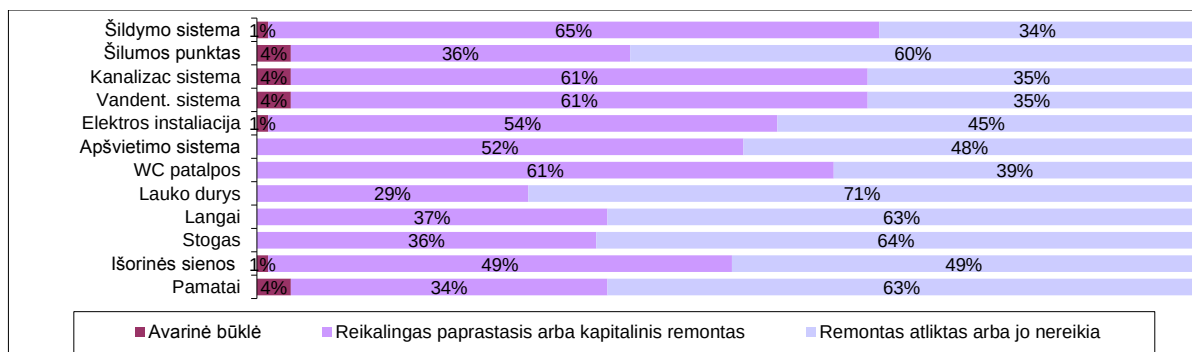
41 pav. Kauno miesto bendrojo ugdymo mokyklų pastatų būklė pagal statinio dalis
