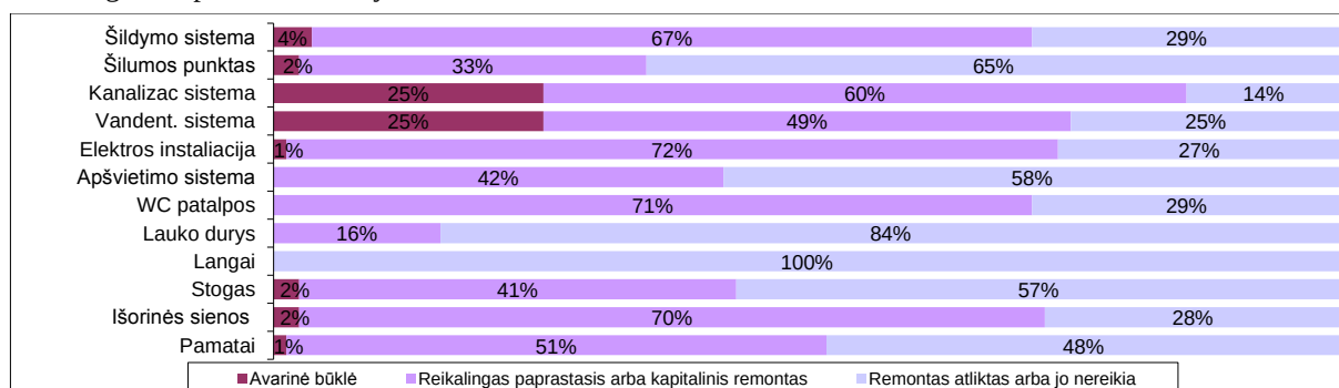
42 pav. Kauno miesto ikimokyklinio ugdymo įstaigų pastatų būklė pagal statinio dalis
