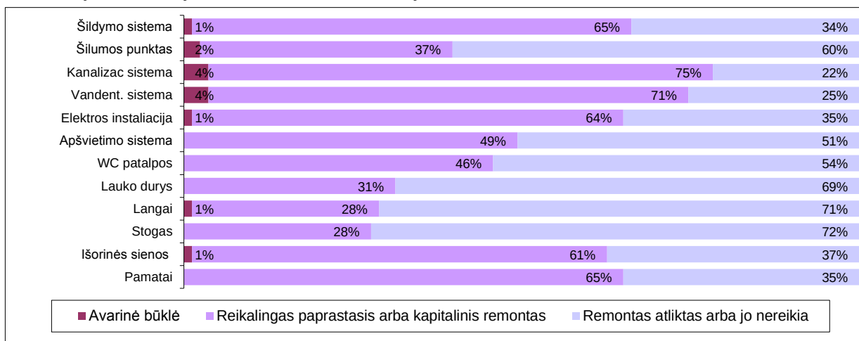
43 pav. Kauno miesto bendrojo ugdymo mokyklų pastatų būklė pagal statinio dalis
