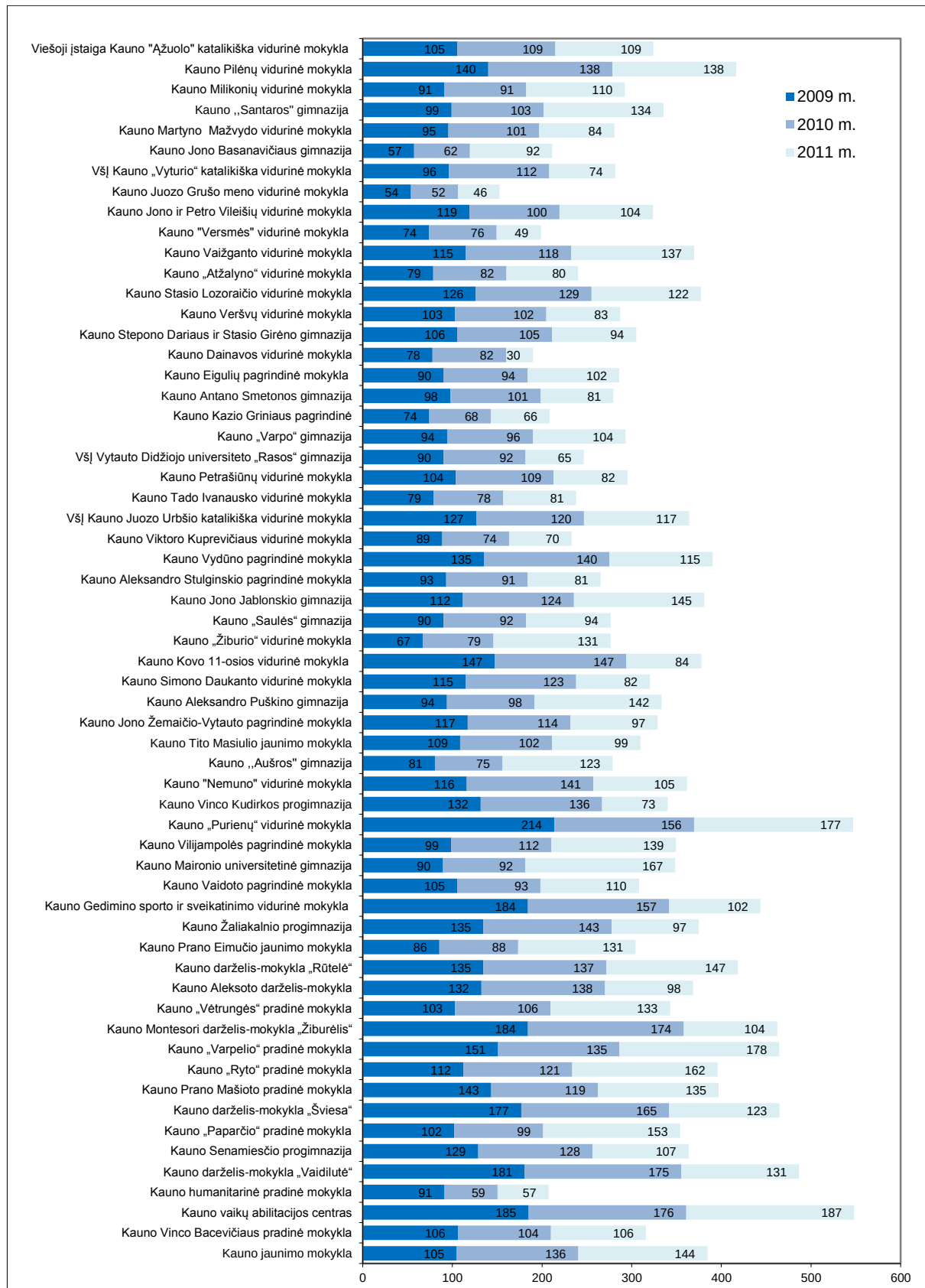
107 pav. Šilumos energijos vartojimo kiekis bendrojo lavinimo mokyklose ( Kwh/m^2 ).
