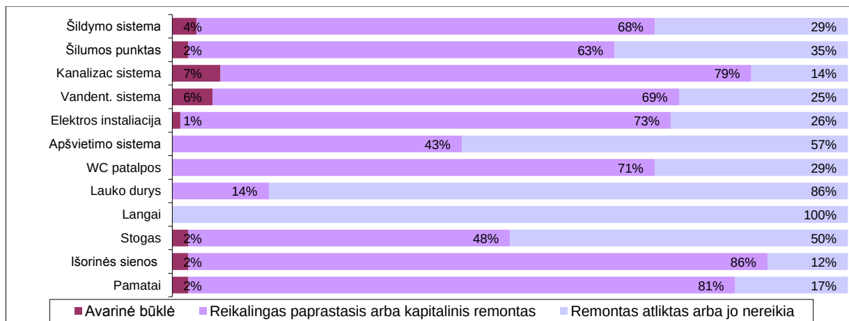
44 pav. Kauno miesto ikimokyklinio ugdymo įstaigų pastatų būklė pagal statinio dalis
