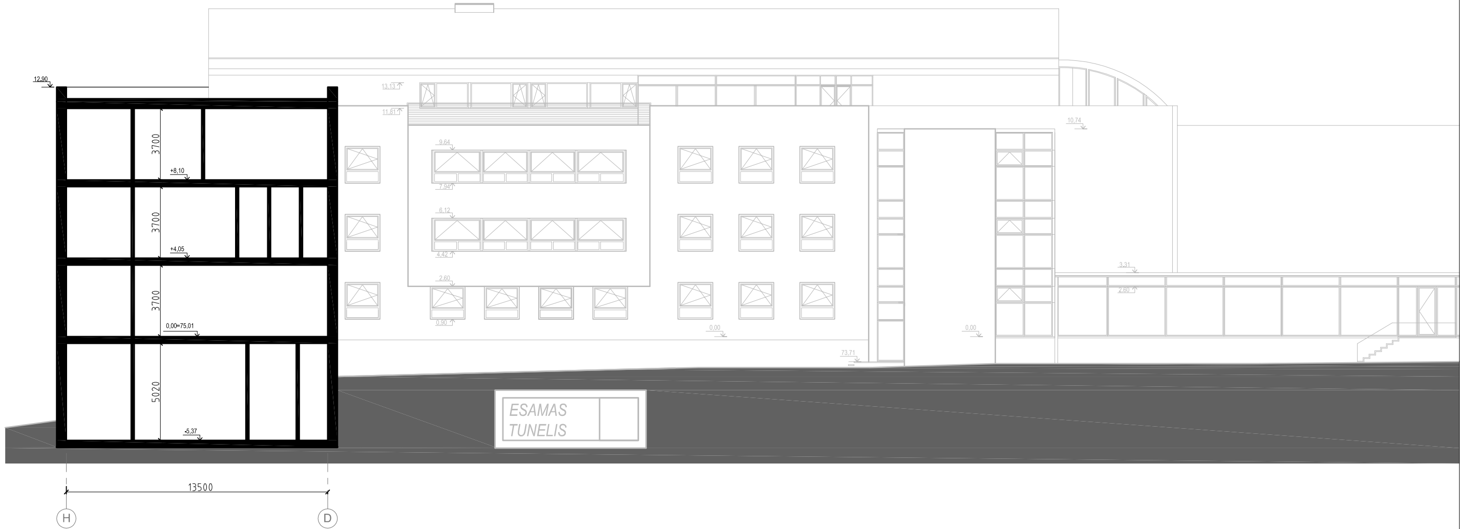
PJŪVIS C-C
