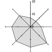
VĖJŲ ROŽĖ
